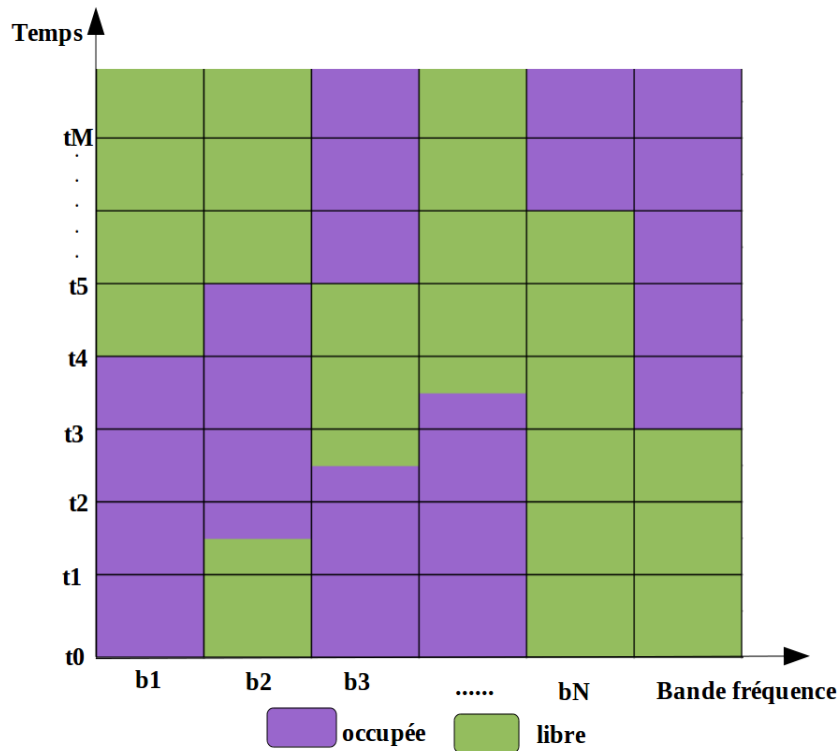
FIGURE 6.3 – Caractérisation du spectre pour le modèle
